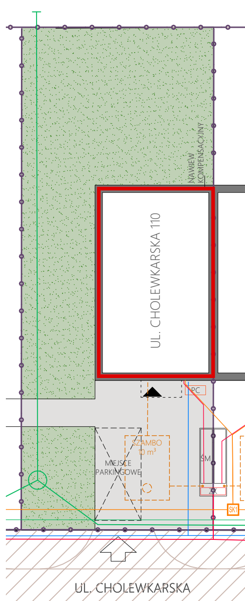
plan sytuacyjny 1:200
